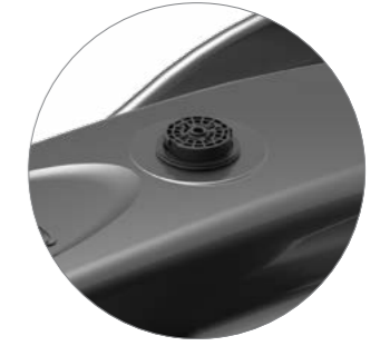
Emplacement pour interfaces ZHAGA © book 18 en partie haute du luminaire (Détecteur de luminosité, noeud de communication radio, etc...) Communication and control reserved area that complies with ZHAGA @ (book 18) connectivity socket. Einbau von Zhaga Standard-Schnittstellen für LED-Module - Buch 18 (Helligkeitssensor, Kommunikationsmodul, usw...)
